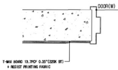
3 DOOR FRAME DETAIL SCALE 1/10
