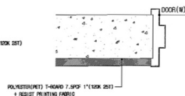
3 DOOR FRAME DETAIL SCALE 1/10
