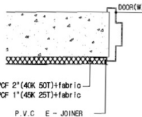
3 DOOR FRAME DETAIL SCALE 1/10
